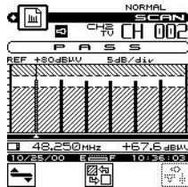
6-Kanal Abnahmemessung
