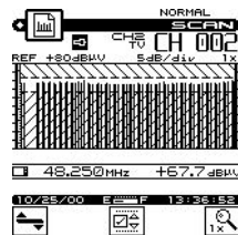
Balayage en fréquences de tous les canaux
