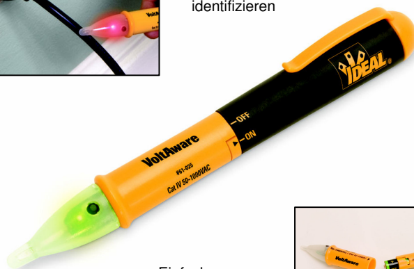
Einfacher Batteriewechsel
