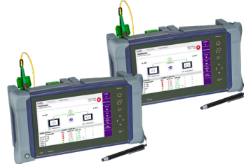
MTS-4000 V2
